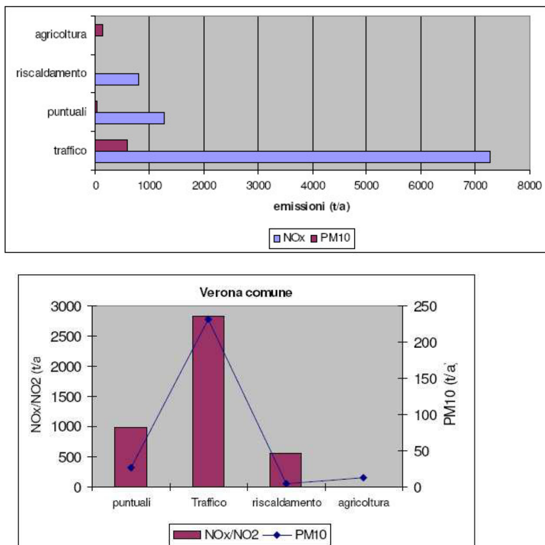
Figura 11: emissioni di ossidi di azoto e polveri sottili dovute alle sorgenti classificate come puntuali (industria), riscaldamento, traffico presenti nel solo comune di Verona –fonte documento UNITN 5
